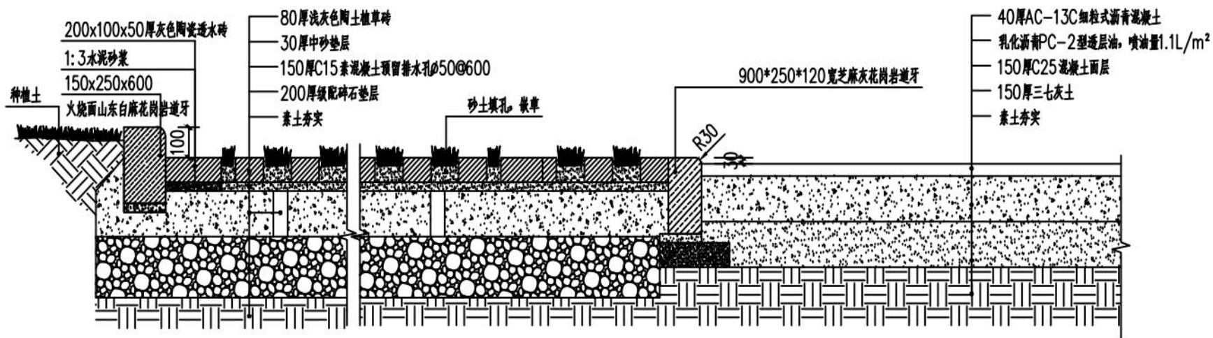
道路做法详图 1:15
